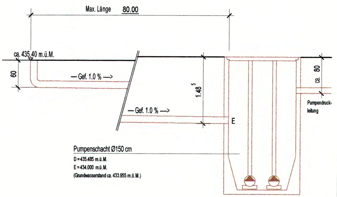
Schemaschnitt Kanalisation 1:50
