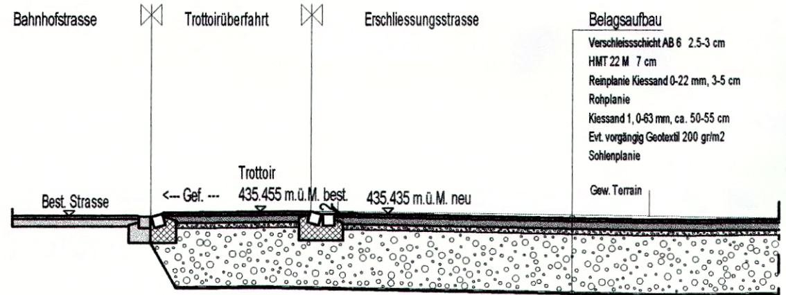
Strassenquerschnitt B-B: Normschnitt Erschliessungsstrasse 1:50
