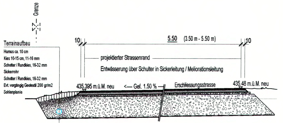
Strassenquerschnitt B-B: Normschnitt Erschliessungsstrasse 1:50
